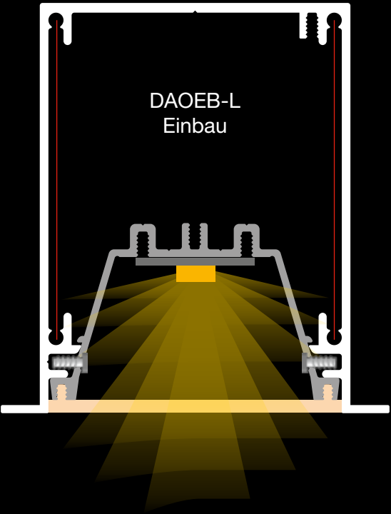
PROFILÜBERSICHT Maßstab 1:1
